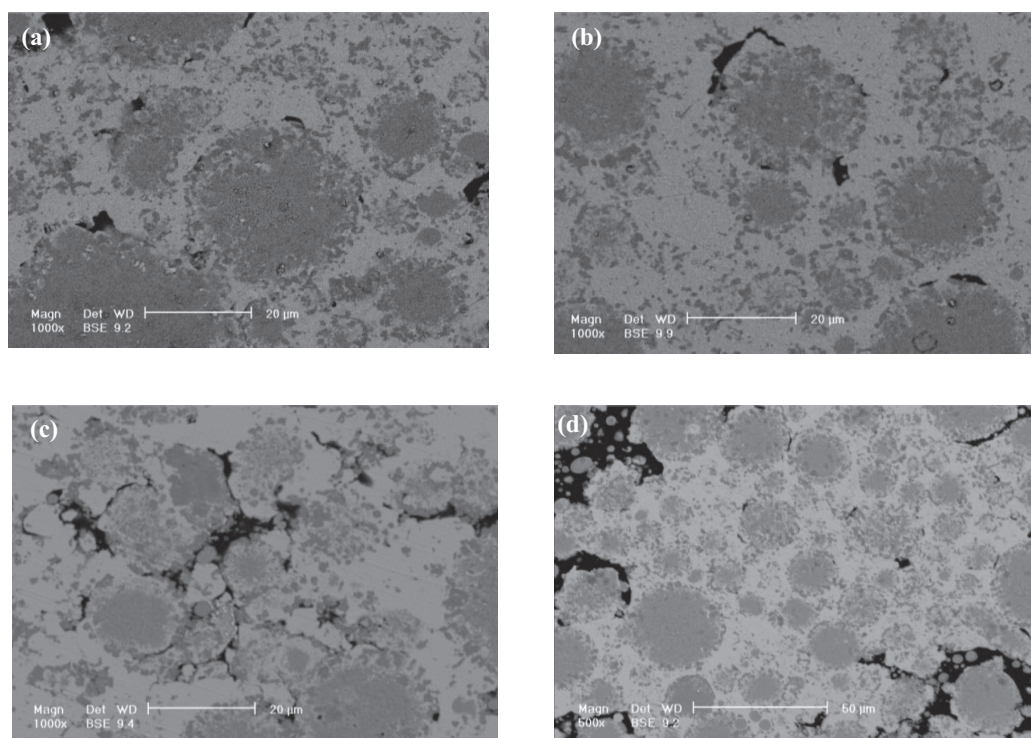
Fig. 4. SEM micrographs of amalgam/ \text{TiO}_2 NPs nanocomposites (a) 0.5 wt. %, (b) 1 wt. %, (c) 2 wt. % and (d) 3 wt. % of \text{TiO}_2 NPs.
