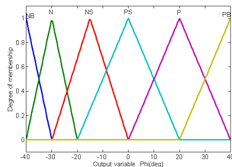
Fig. 12. MF( \phi )
