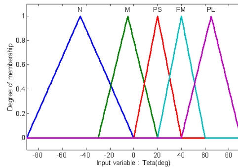
Fig. 11. MF( \theta )
